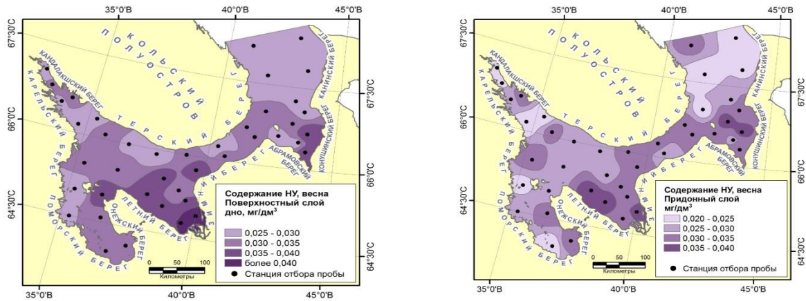
Рис. 4. Распределение средней концентрации НУ в поверхностном (а) и придонном (б) слоях вод Белого моря в весенние периоды 2001-2016 гг.
