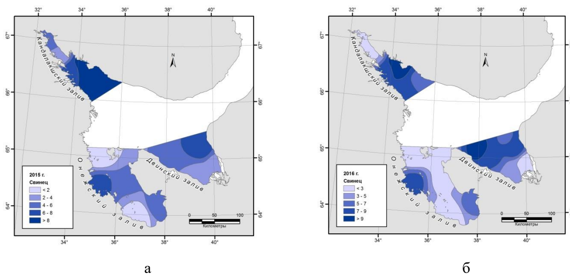
Рис.14. Распределение свинца (мг/кг) в донных отложениях в Двинском, Онежском и Кандалакшском заливах в 2015 (а) и 2016 (б) гг.
