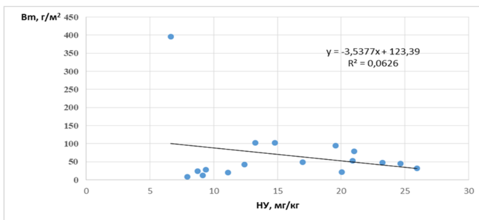
Рис. 19. Зависимость биомассы макрозообентоса Двинского залива Белого моря от содержания НУ в донных отложениях ( r = -0,250 ).
