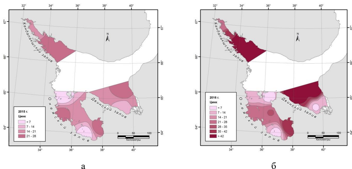
Рис. 17. Распределение цинка (мг/кг) в донных отложениях в Двинском, Онежском и Кандалакшском заливах в 2015 (а) и 2016 (б) гг.
