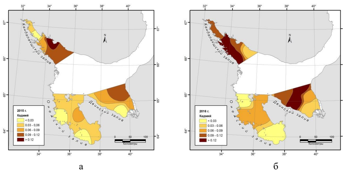
Рис. 15. Распределение кадмия (мг/кг) в донных отложениях в Двинском, Онежском и Кандалакшском заливах в 2015 (а) и 2016 (б) гг.
