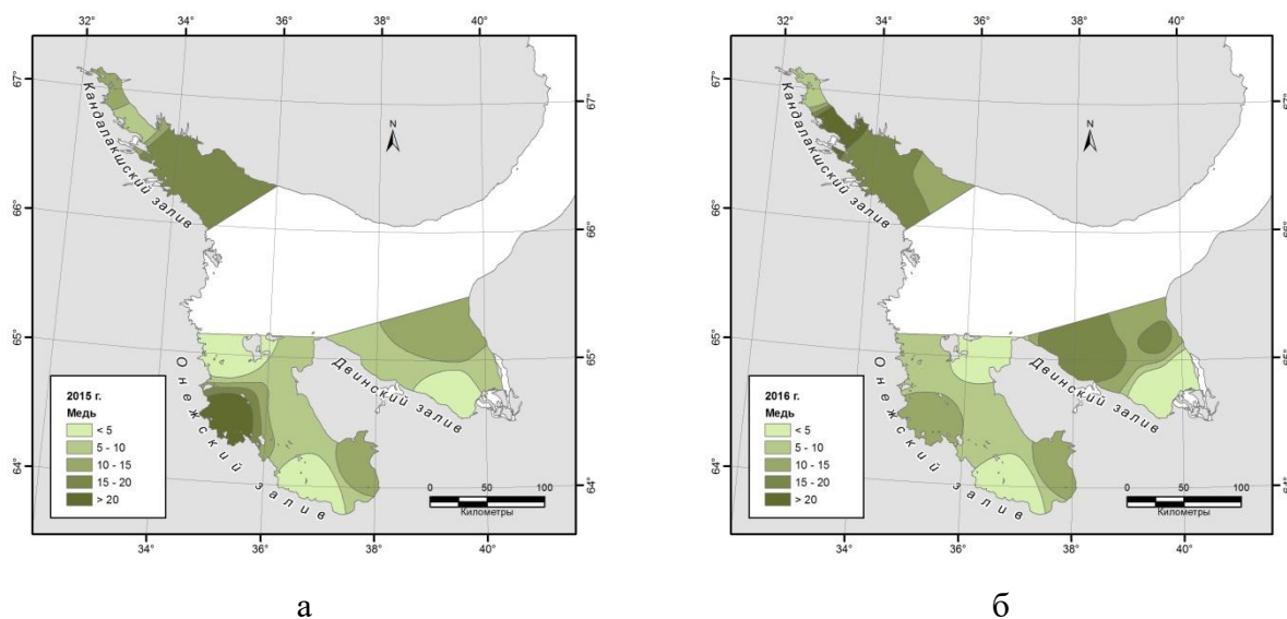
Рис. 16. Распределение меди (мг/кг) в донных отложениях в Двинском, Онежском и Кандалакшском заливах в 2015 (а) и 2016 (б) гг.
