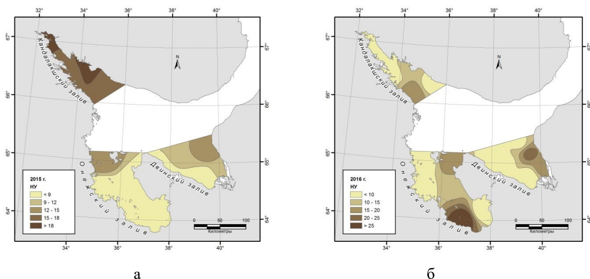
Рис. 13. Распределение нефтепродуктов (мг/кг) в донных отложениях в Двинском, Онежском и Кандалакшском заливах в 2015 (а) и 2016 (б) гг.
