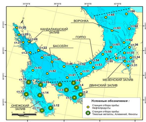
Рис. 1. - Карта-схема расположения комплексных станций в Белом море.
