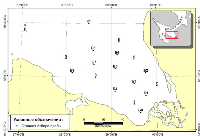
Рис. 3. - Станции отбора проб макрозообентоса и ДО в Двинском заливе Белого моря в 2016 г.
