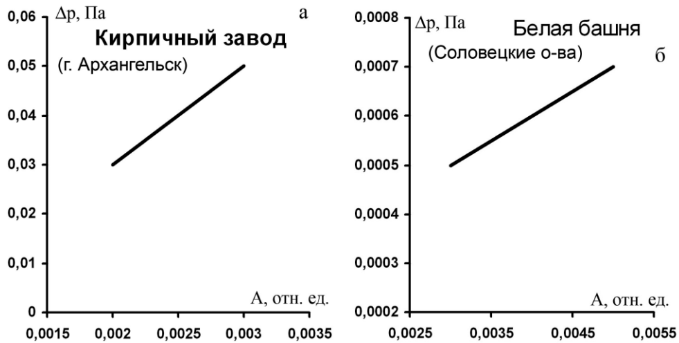
Рисунок 2 – Калибровочные кривые для разных типов инженерных сооружений
