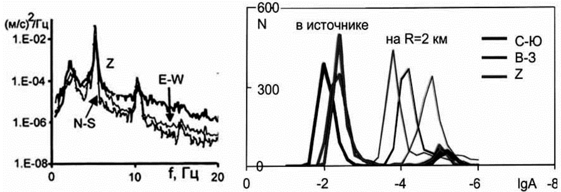
Рисунок 1 – Типичные спектры мощности микросейсм вблизи источника и распределения значений амплитуд для двух точек наблюдения вблизи источника и на расстоянии 2 км
