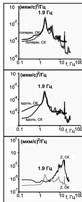
Рисунок 3 – Спектры записей в аварийном жилом доме (СК) и в соседнем целом (ОК) (этот же проект) на 9 бл этажах
