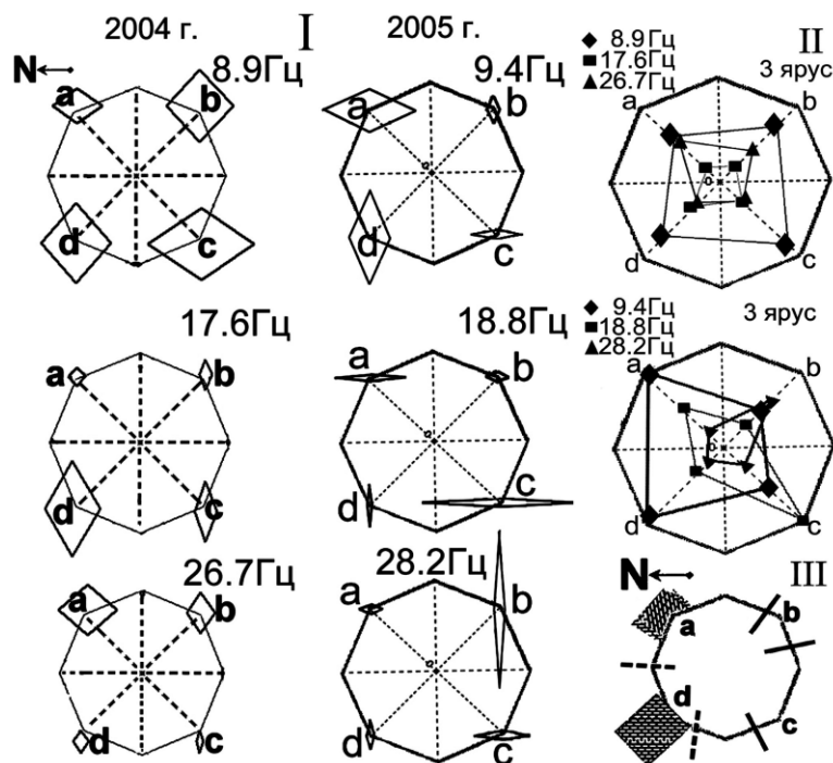
Рисунок 4 – Диаграммы-ромбы (I), построенные на основании полярных диаграмм амплитуд разных мод собственных колебаний башни в горизонтальной плоскости (II) для набора точек и частот, данные 2004 – 2005 гг.; план-схема по результатам обследования состояния Белой башни (III), нанесены трещины – развивающиеся (сплошная линия) и новые (пунктир)
