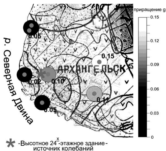
Рисунок 6 – Карта ускорений (в долях g) территории г. Архангельска
